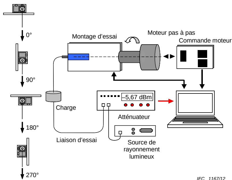
Figure 4 – Montage de l'équipement par la méthode B pour des interfaces Rx et des récepteurs optiques
