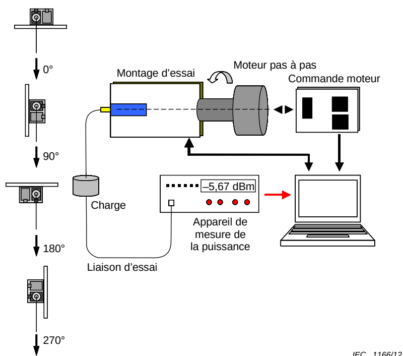
Figure 3 – Montage de l'équipement par la méthode B pour des interfaces Tx
