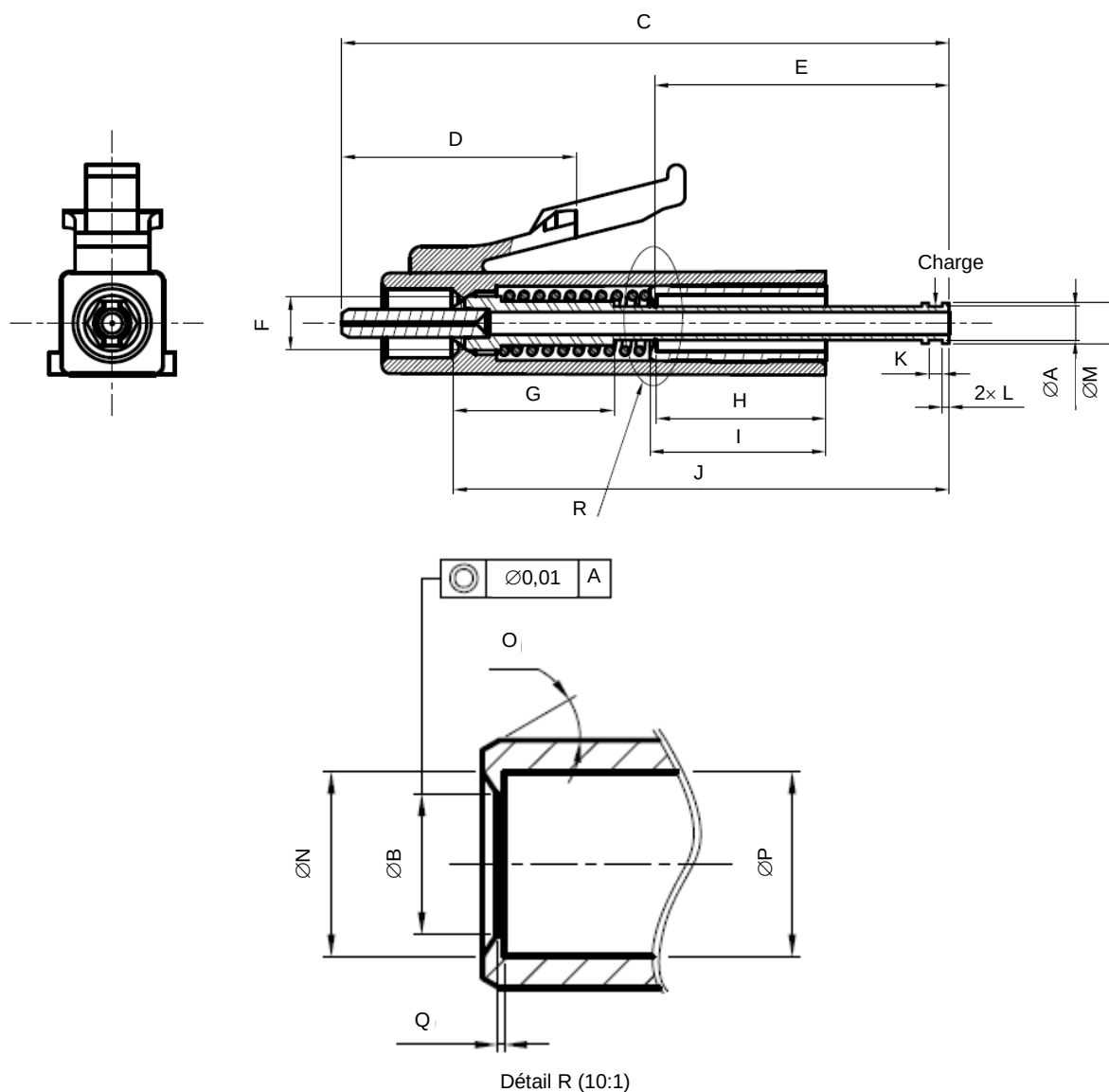
Figure C.1 – Interface de cordon d'essai pour perturbations d'origine mécanique
