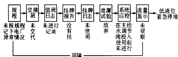
图3 核电厂 SG 人因事件屏障分析图
