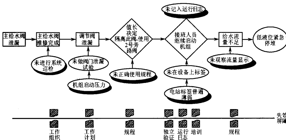
图2 核电厂 SG 人因事件 E &amp; CF 图
