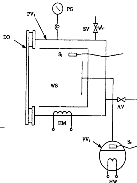
图 D2 双容器型
